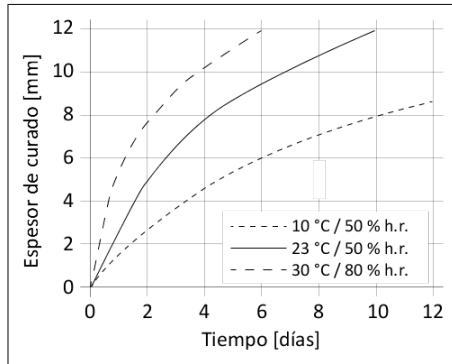
Diagrama 1: Velocidad de curado SikaTack® Panel
